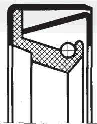
WCL se sevrženou gumovou manžetou
