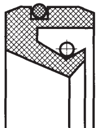
WEPO PTFE provedení s jistícím O-KROUŽKEM, který funguje jako pouzdrové těsnění
