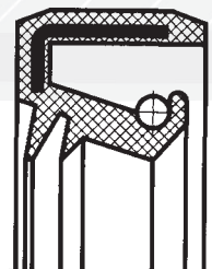
WAV se dvěma prachovými břity
