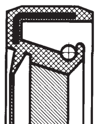
WAB se šroubovicí pro zpětnou dopravu doleva a šroubo - vicí na prachovém břitu
