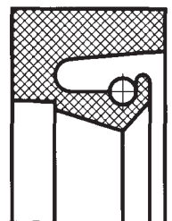
WEP PTFE provedení
