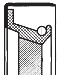
WBH se šroubovicí pro zpětnou dopravu doprava
