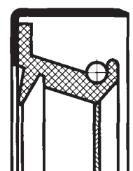
WBF se šroubovicemi se střídavě levým a pravým stoupáním s prachovým břity
