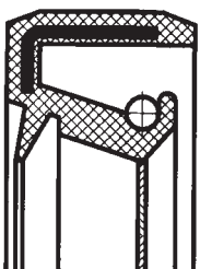
WAF se dvěma prachovými břity
