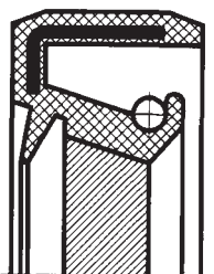
WAU se šroubovicí pro zpětnou dopravu doprava a pracho vým břitem
