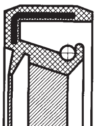
WAE se šroubovicí pro zpětnou dopravu doprava a šroubo - vicí na prachovém břitu
