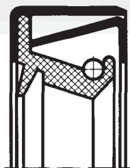
WCR se sevrženou gumovou manžetou a prachovým břitem
