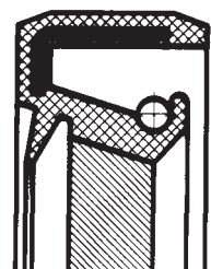
WAT se šroubovicí pro zpětnou dopravu doleva a pracho - vým břitem
