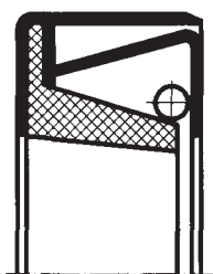
WCP se sevrženou PTFE manžetou
