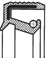
WAG s drážkami na vnějším plášti a prachovým břitem
