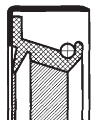
WBE se šroubovicí pro zpětnou dopravu doprava a šroubo - vicí na prachovém břitu
