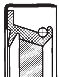
WBU se šroubovicí pro zpětnou dopravu doprava a pracho - vým břitem
